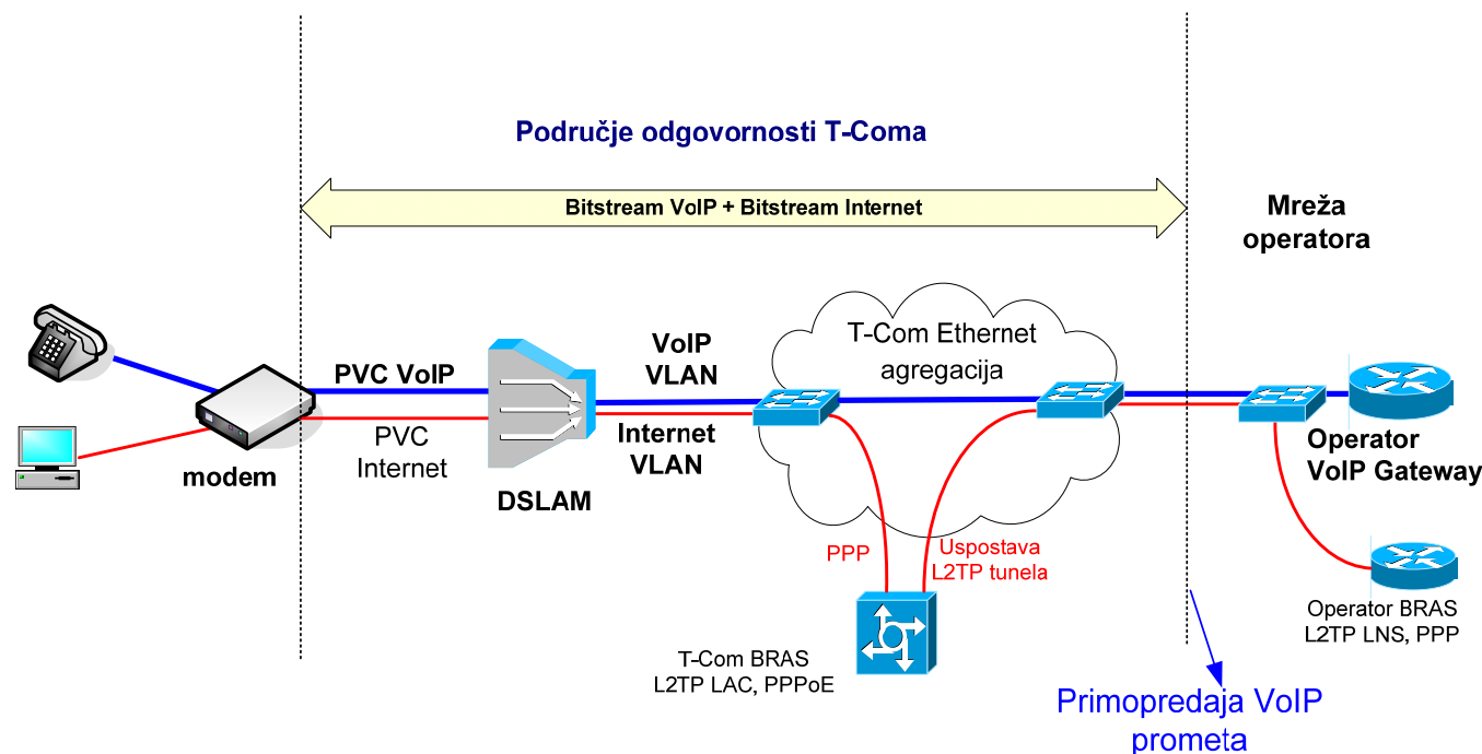
Slika 8. Realizacija posebnog virtualnog kanala za VoIP uslugu preko ADSL pristupa
