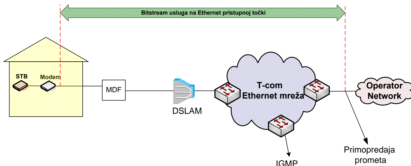
Slika 20. IPTV usluga na Ethernet razini putem ADSL tehnologije u slučaju kada Krajnji korisnik ostvaruje Osnovni pristup mreži putem usluge Operatora korisnika
