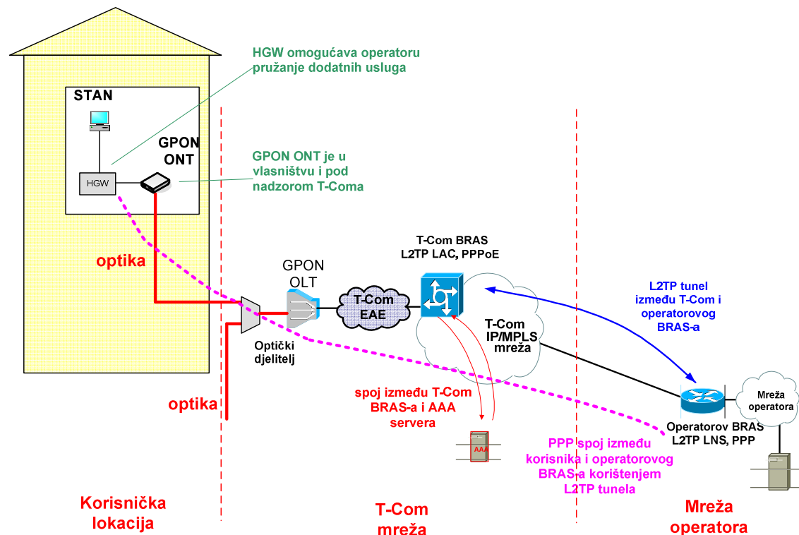
Slika 2. Način realizacije usluge veleprodajnog širokopojsnog pristupa za Internet uslugu na temelju FTTH tehnologije na IP razini
