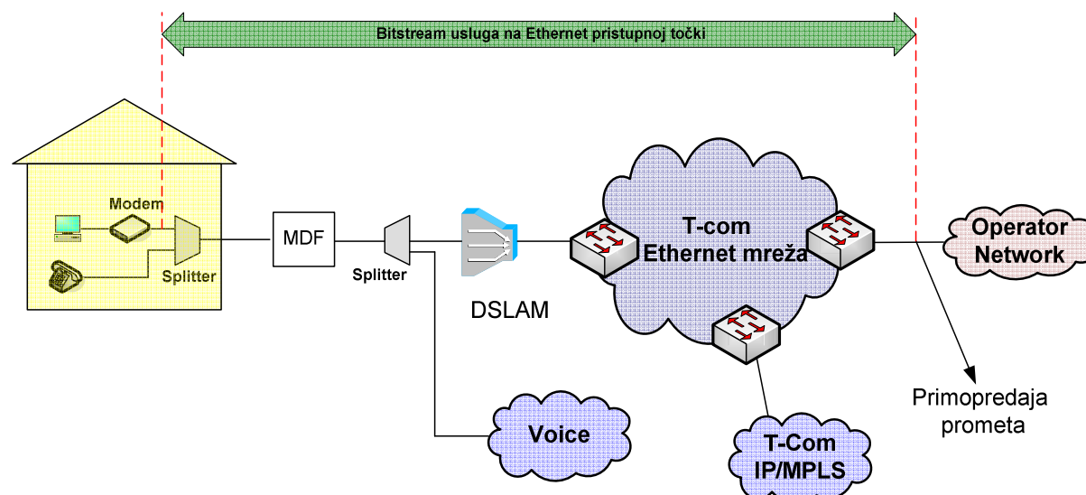
Slika 10. Veleprodajni širokopolasni pristup za pružanje VoIP usluge na Ethernet razini u slučaju kada Krajnji korisnik ostvaruje Osnovni pristup mreži putem usluge T-Coma
