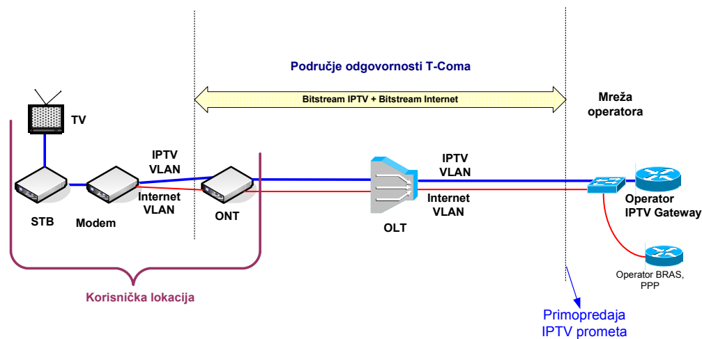
Slika 21. Veleprodajni širokopolasni pristup za pružanje IPTV usluge preko FTTH pristupa (GPON) na OLT razini
