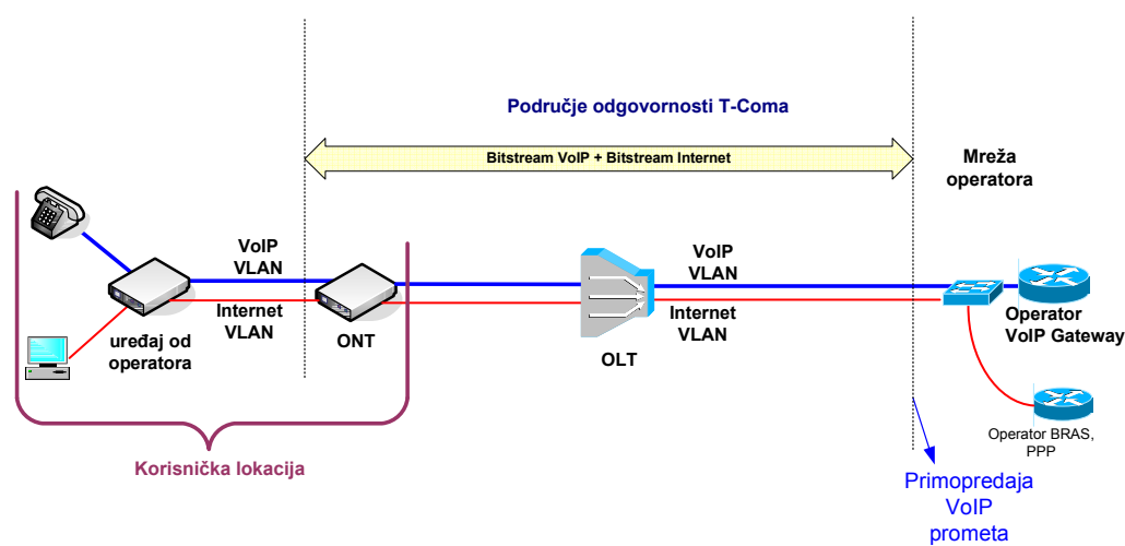
Slika 14. Veleprodajni širokopojasni pristup za pružanje VoIP usluge preko FTTH pristupa (GPON) na OLT razini
