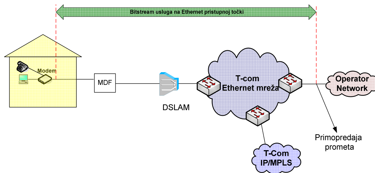
Slika 11. Veleprodajni širokopolasni pristup za pružanje VoIP usluge na Ethernet razini u slučaju kada Krajnji korisnik ostvaruje Osnovni pristup mreži putem usluge Operatora korisnika
