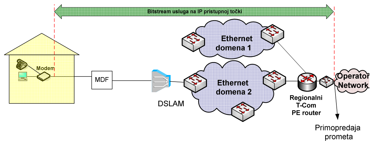
Slika 13. Veleprodajni širokopojasni pristup za pružanje VoIP usluge na IP razini u slučaju kada Krajnji korisnik ostvaruje Osnovni pristup mreži putem usluge Operatora korisnika
