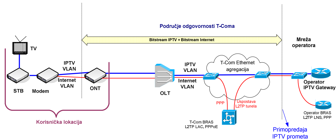
Slika 18. Realizacija posebnog virtualnog kanala za IPTV uslugu preko FTTH pristupa (GPON)
