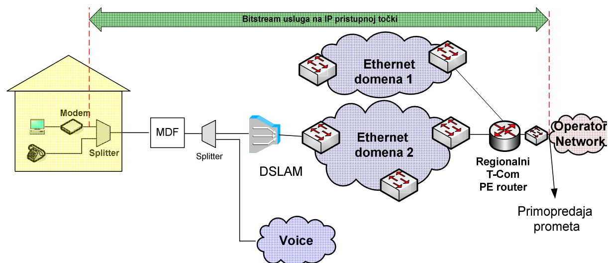
Slika 12. Veleprodajni širokopolasni pristup za pružanje VoIP usluge na IP razini u slučaju kada Krajnji korisnik ostvaruje Osnovni pristup mreži putem usluge T-Coma
