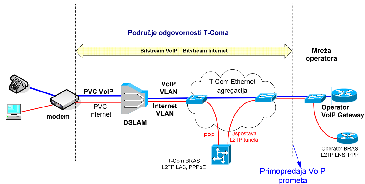
Slika 8. Realizacija posebnog virtualnog kanala za VoIP uslugu preko ADSL/VDSL pristupa (kod VDSL pristupa između modema i DSLAM-a koristi se odgovarajući VLAN)
