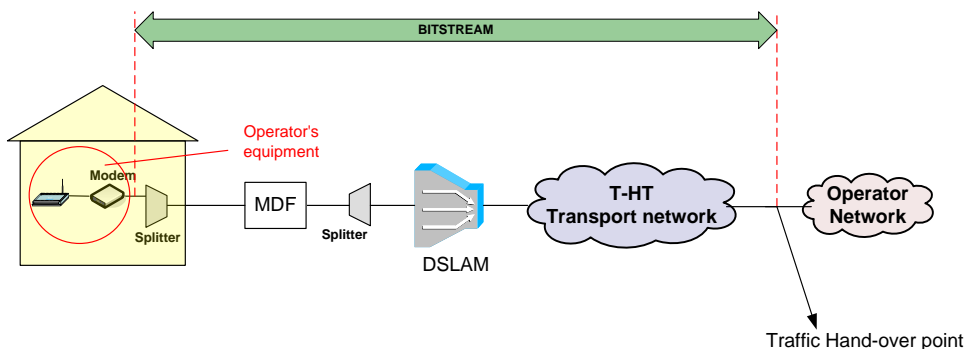
Slika 31. Koncept posebnog virtualnog kanala za Podatkovnu uslugu
