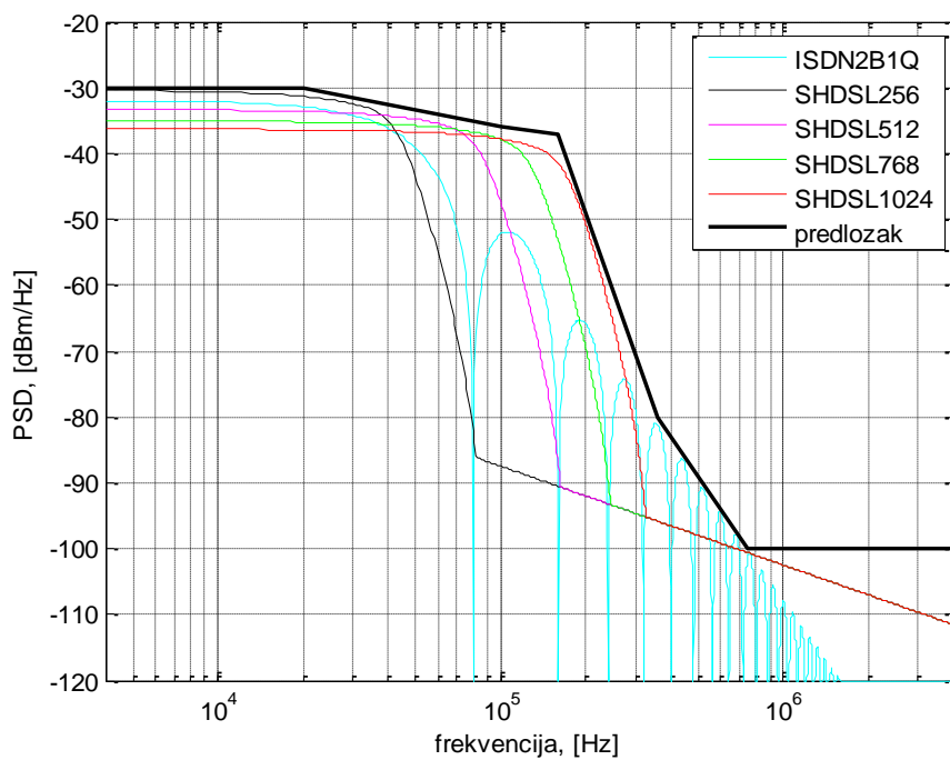
Slika 5.6.5 Frekvencijski predložak za odlazni smjer prijenosa (duge pretplatničke linije) za ADSL preko POTS (aneks A).
