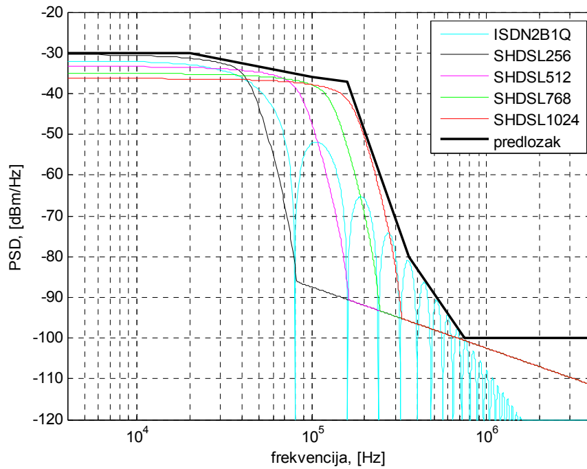
Slika 5.6.5 Frekvencijski predložak za odlazni smjer prijensa (duge pretplatničke linije) za ADSL preko POTS (aneks A).
