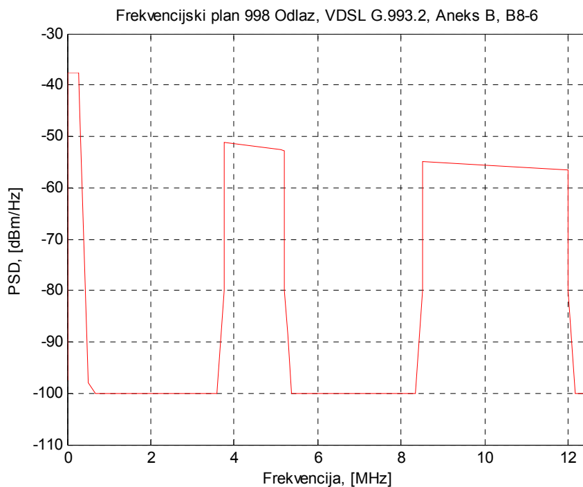
Slika 5.6.2 Frekvencijski predložak za odlazni smjer prijena za VDSL2, frekvencijski plan 998, B8-6
