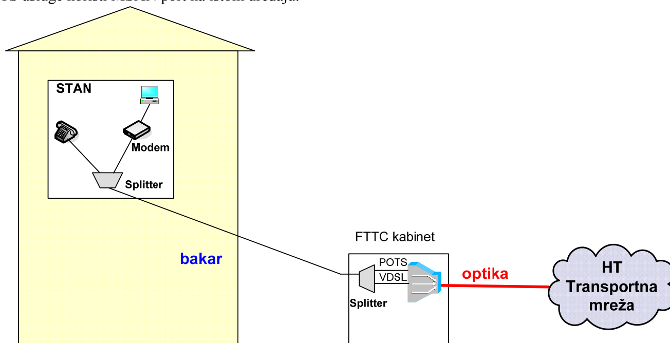
Slika 30. Način realizacije FTTC koncepta u pristupnoj mreži
