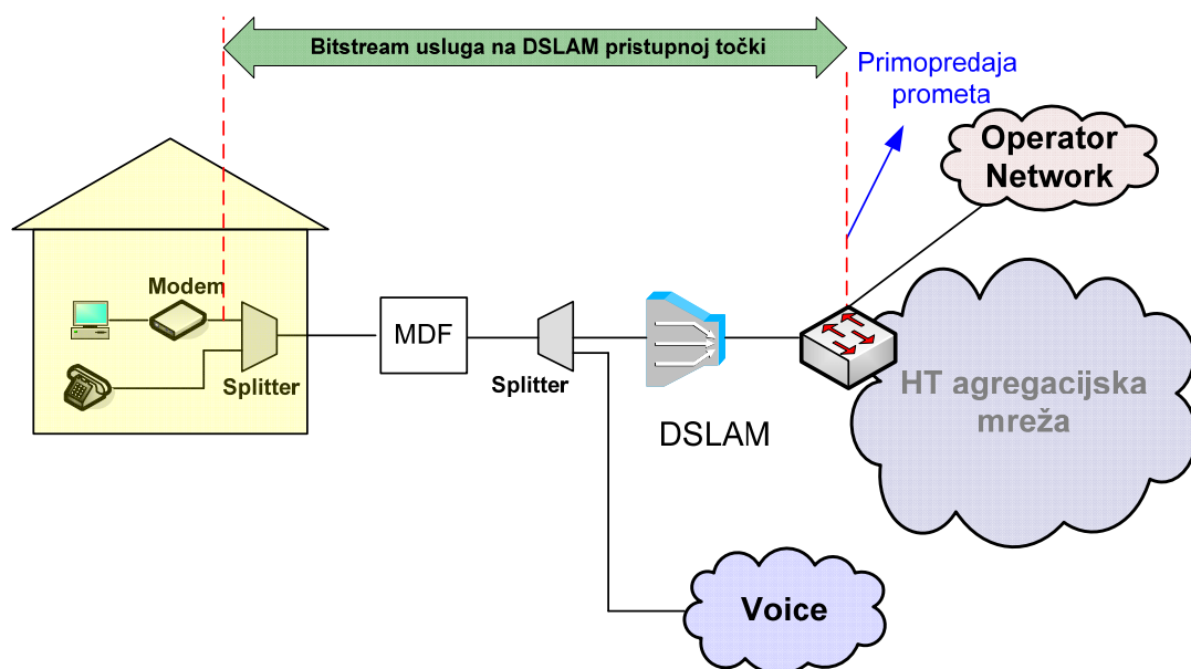
Slika 7. Veleprodajni širokopojasni pristup za pružanje Internet usluge na DSLAM razini u slučaju kada krajnji korisnik ostvaruje Osnovni pristup mreži putem usluge HT-a
