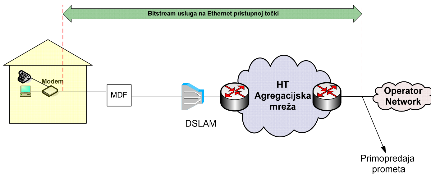
Slika 14. Veleprodajni širokopojsni pristup za pružanje VoIP usluge na Ethernet razini u slučaju kada krajnji korisnik ostvaruje Osnovni pristup mreži putem usluge HT-a
