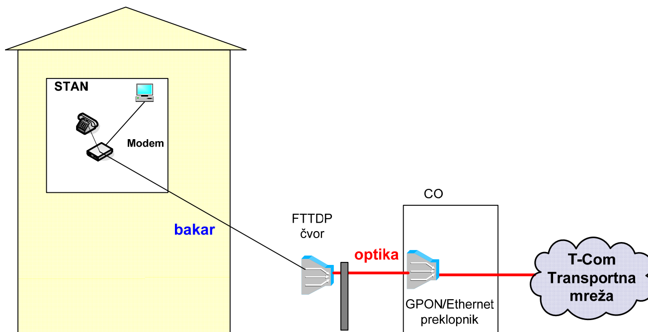
Slika 35. Način realizacije FTTDP koncepta u pristupnoj mreži
