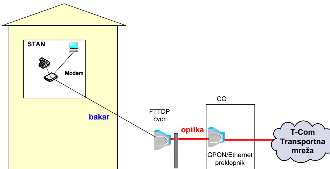
Slika 36. Način realizacije FTTDP koncepta u pristupnoj mreži
