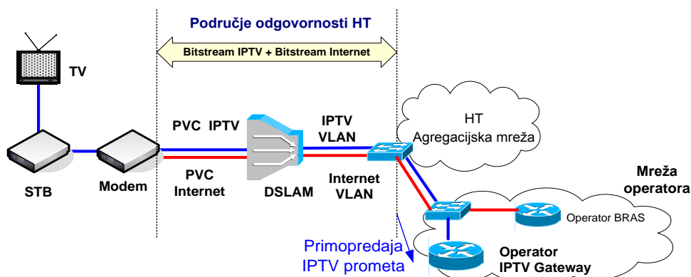
Slika 27. Veleprodajni širokopolasni pristup za pružanje IPTV usluge preko ADSL/VDSL pristupa na DSLAM razini
