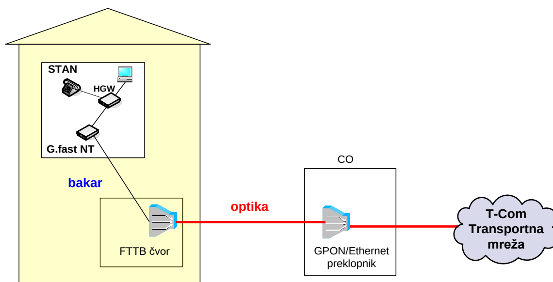
Slika 35a. Način realizacije FTTB koncepta sa G.fast tehnologijom u pristupnoj mreži
