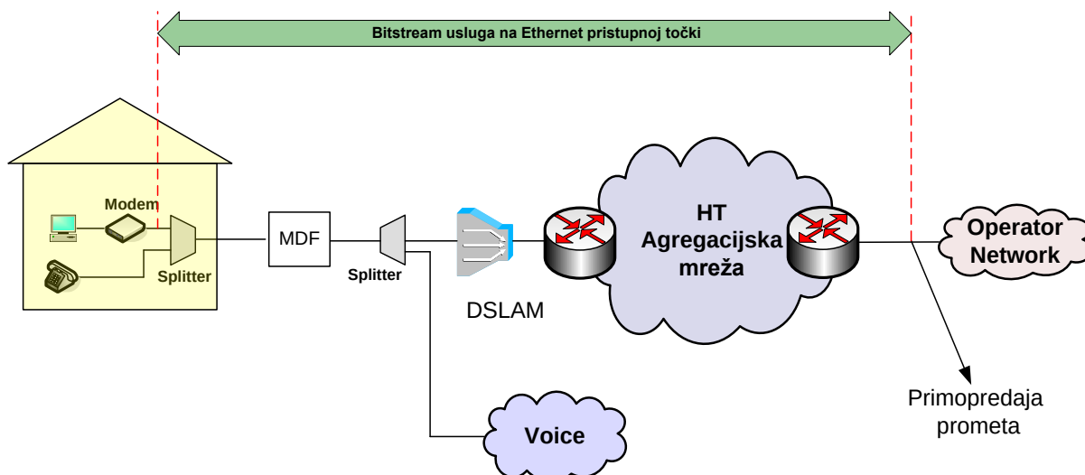
Slika 14. Veleprodajni širokopojasni pristup za pružanje VoIP usluge na Ethernet razini u slučaju kada krajnji korisnik ostvaruje Osnovni pristup mreži putem usluge HT-a
