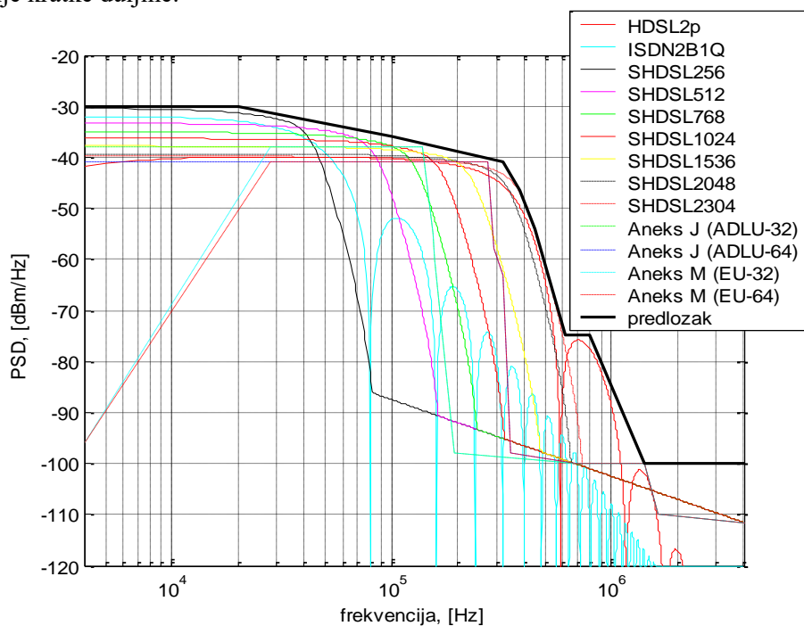
Slika 5.67.1 Frekvencijski predložak za odlazni smjer prijenosa (kratke pretplatničke linije).
