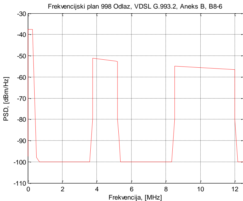
Slika 5.67.2 Frekvencijski predložak za odlazni smjer prijenosa za VDSL2, frekvencijski plan 998, B8-6
