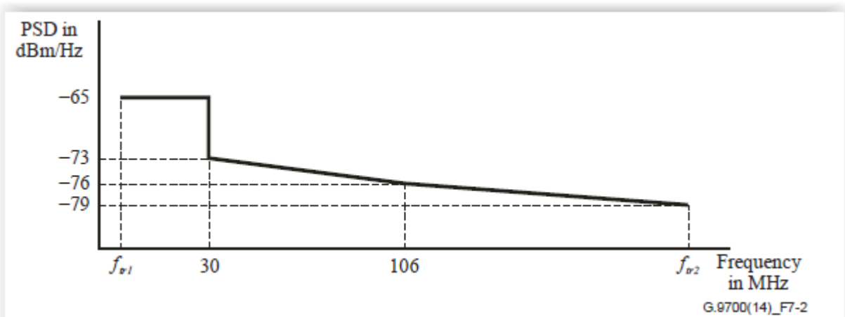
Slika 4.9.2 - Maska PSD za G.fast 212 MHz profil
