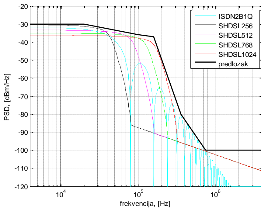
Slika 5.67.5-7 Frekvencijski predložak za odlazni smjer prijenosa (duge pretplatničke linije) za ADSL preko POTS (aneks A).
