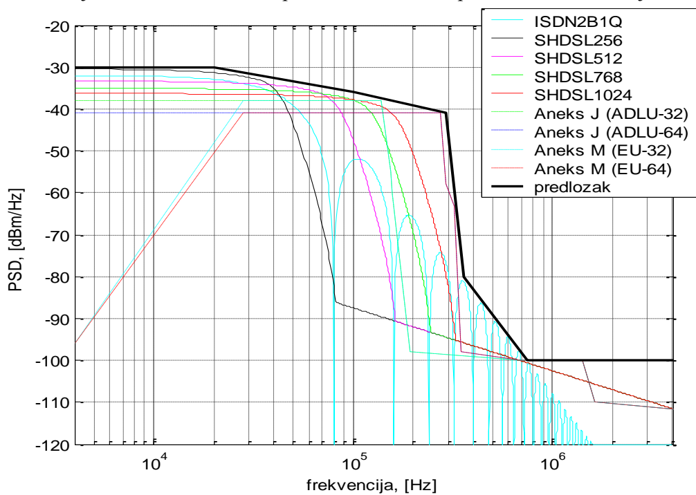
Slika 5.67.4-6 Frekvencijski predložak za odlazni smjer prijenosa (duge pretplatničke linije) za ADSL preko ISDN (aneks B).
