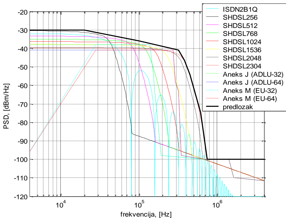
Slika 5.67.3-5 Frekvencijski predložak za odlazni smjer prijenosa (pretplatničke linije srednje duljine).
