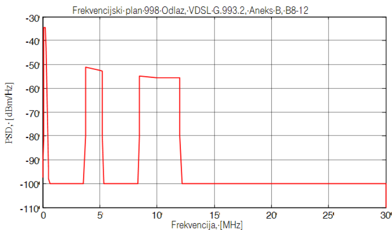
Slika 5.67.3 Frekvijski predložak za odlazni smjer prijenosa za VDSL2, frekvijski plan 998, B8-12
