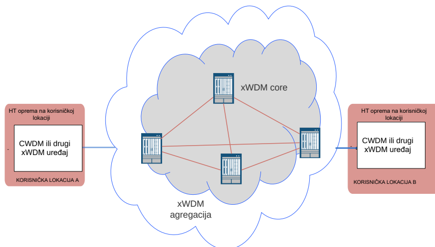
Slika 2. Načelan prikaz E2E realizacije xWDM voda
