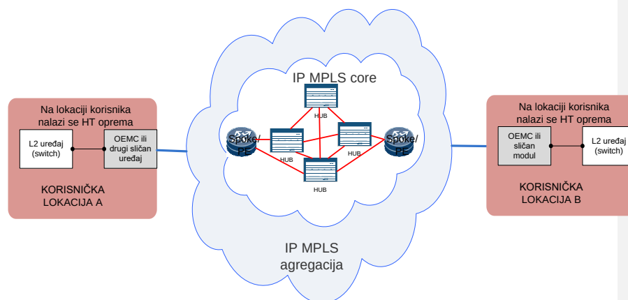
Slika 1. Načelan prikaz E2E realizacije Ethernet voda
