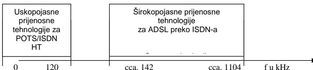
Slika 1. Frekvencijski opseg za uskopojasne i širokopojasne prijenosne tehnologije
