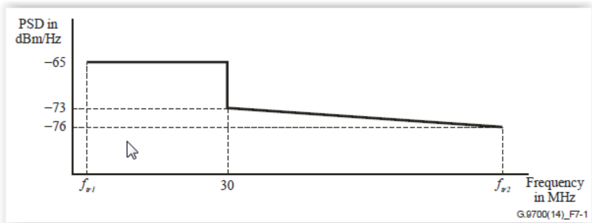
Slika 4.9.1 - Maska PSD za G.fast 106 MHz profil
