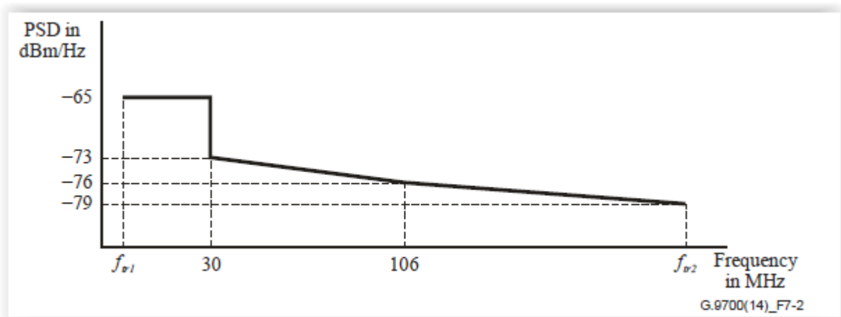
Slika 4.9.2 - Maska PSD za G.fast 212 MHz profil*
