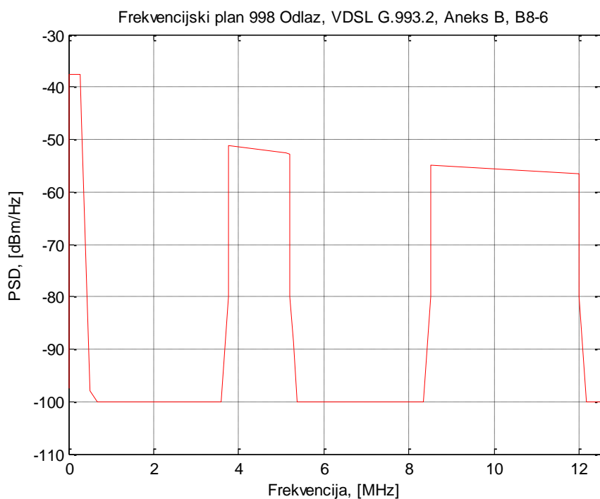
Slika 5.7.2 Frekvenjski predložak za odlazni smjer prijenosa za VDSL2, frekvenjski plan 998, B8-6
