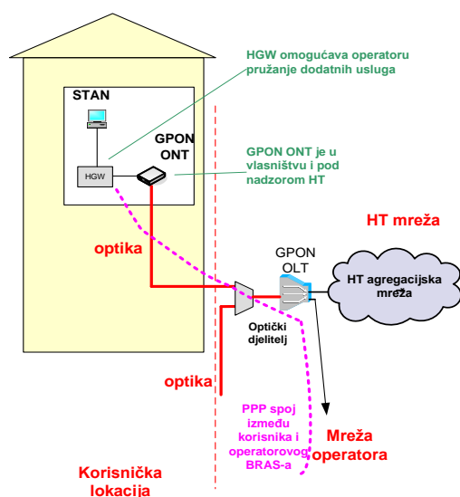
Slika 6. Način realizacije usluge veleprodajnog širokopolasnog pristupa za Internet uslugu na temelju FTTH rješenja na OLT razini
