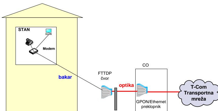
Slika 36. Način realizacije FTTP koncepta sa VDSL17a tehnologijom u pristupnoj mreži
