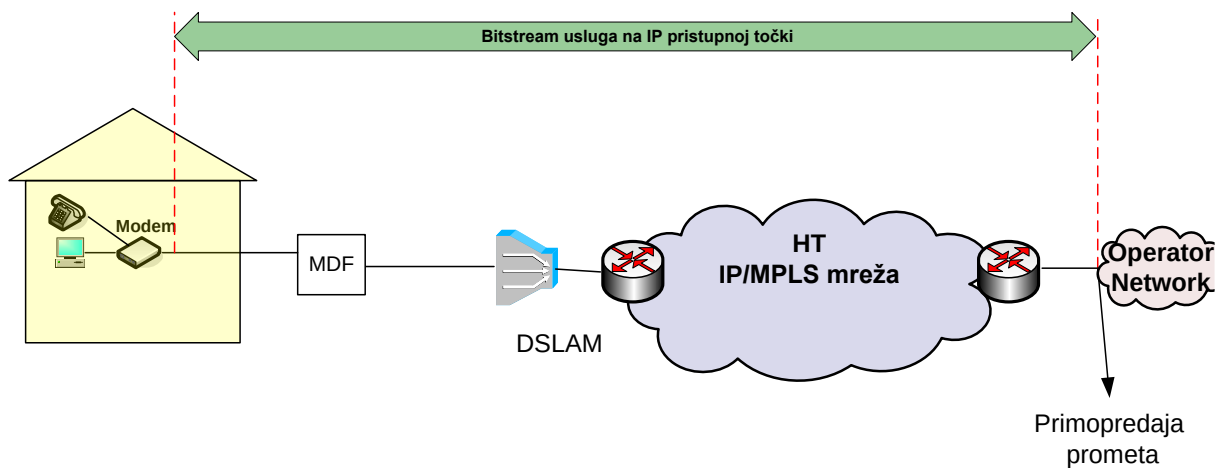
Slika 16. Veleprodajni širokopojasni pristup za pružanje VoIP usluge na IP razini u slučaju kada krajnji korisnik ostvaruje Osnovni pristup mreži putem usluge HT-a
